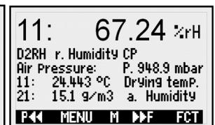
Sensor display
